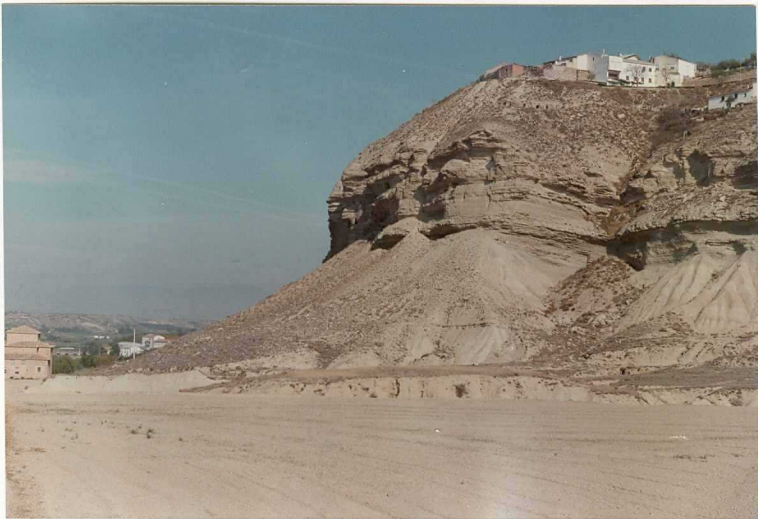
FOTO 9011.- Panorámica del contacto entre las unidades (16). Margas con niveles de yeso, y la (17). Yesos de los Arcos, en la localidad de Lerin.
